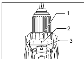
1. Anillo de ajuste 2. Graduación 3. Puntero
