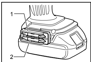
1. Portabrocas 2. Punta
